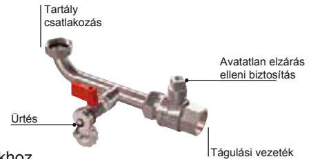
Tágulási vezeték
